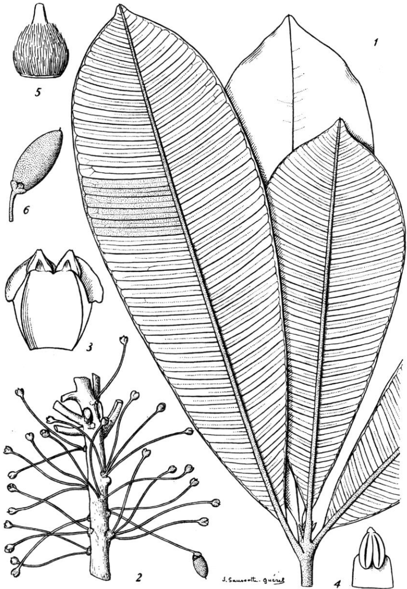
Pl. 1. — Englerophytum somiferanum A. Aubr. : 1, rameau feuillé \times 2/3 ; 2, inflorescence \times 2/3 ; 3, fragment de corolle \times 8 ; 4, anthère vue de l'extérieur \times 8 ; 5, pistil \times 8 ; 6, jeune fruit, gr. nat.
